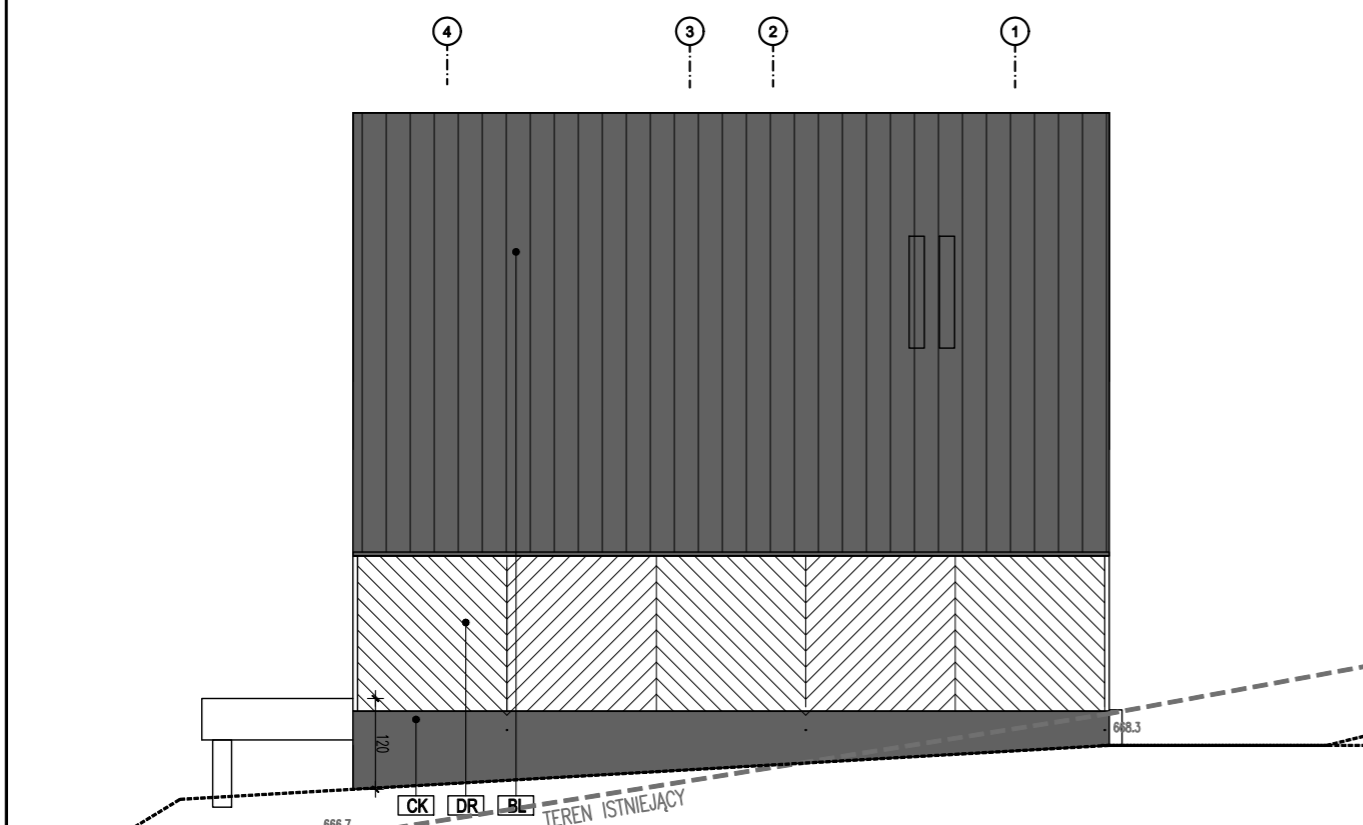
ELEWACJA PÓLNOCCO - WSCHODNIA
