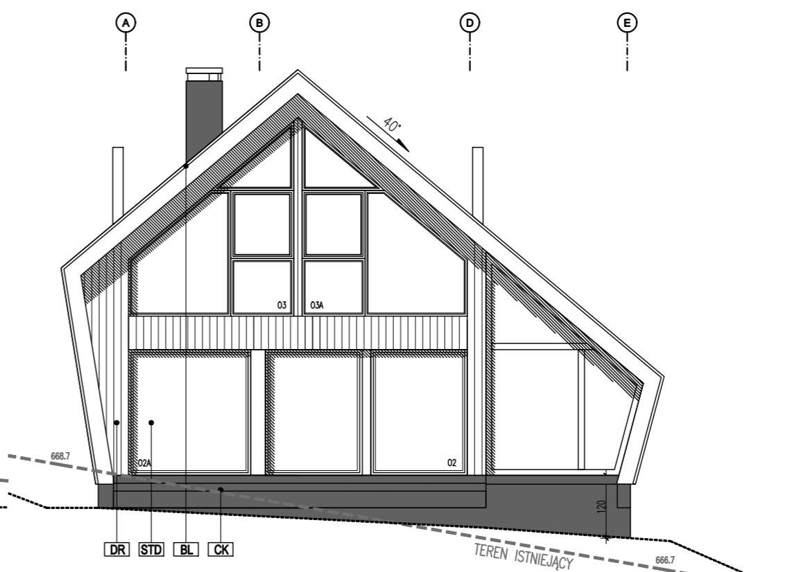
ELEWACJA POŁUDNIOWO - WSCHODNIA
