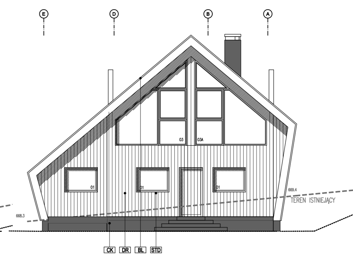
ELEWACJA PÓLNOCCO - ZACHODNIA
